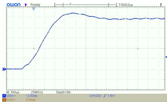
Рис. 16. Переходный процесс при уставке напряжения 5 В Fig. 16. Transient process at a voltage setting of 5 V
