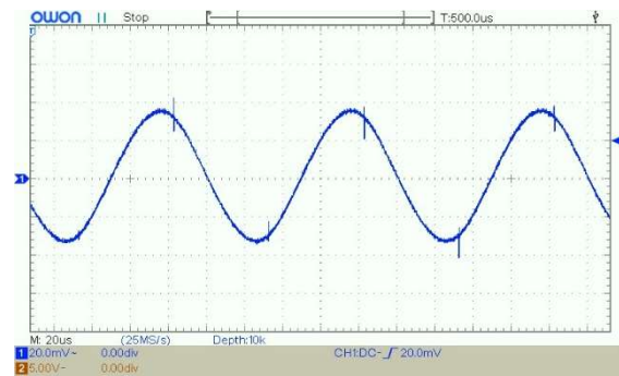
Рис. 17. Пульсации при уставке напряжения 5 В Fig. 17. Ripple at 5 V voltage setting
