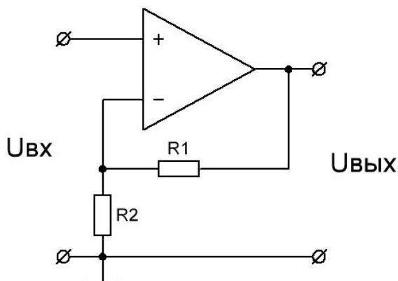
Рис. 9. Схема неинвертирующего усилителя Fig. 9. Non-inverting amplifier circuit
